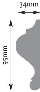
PD 48 3m Length
